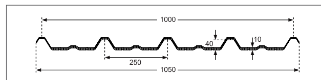
GT40 10 mm U-waarde 2,8 W/m 2 K
