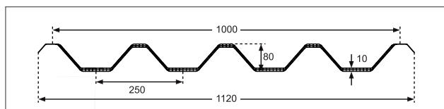
GT80 10 mm U-waarde 2,8 W/m 2 K
