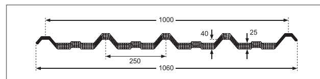
GT40 25 mm U-waarde 1,4 W/m 2 K
