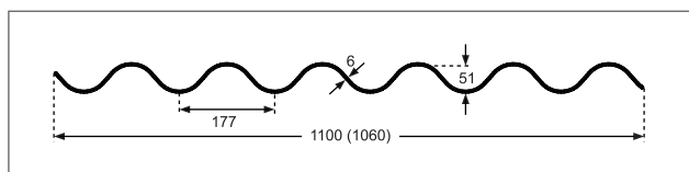
177/51 6 mm U-waarde 3,3 W/m 2 K
