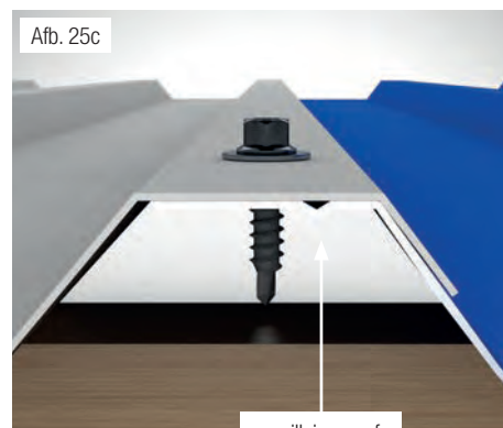
damwandprofiel 35/1035
